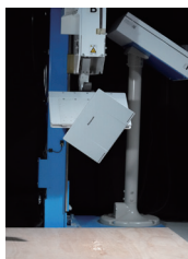
76cm落下※(26方向/動作時)
