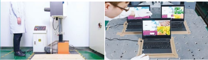
各面、辺、角の26方向から76cm落下テスト
